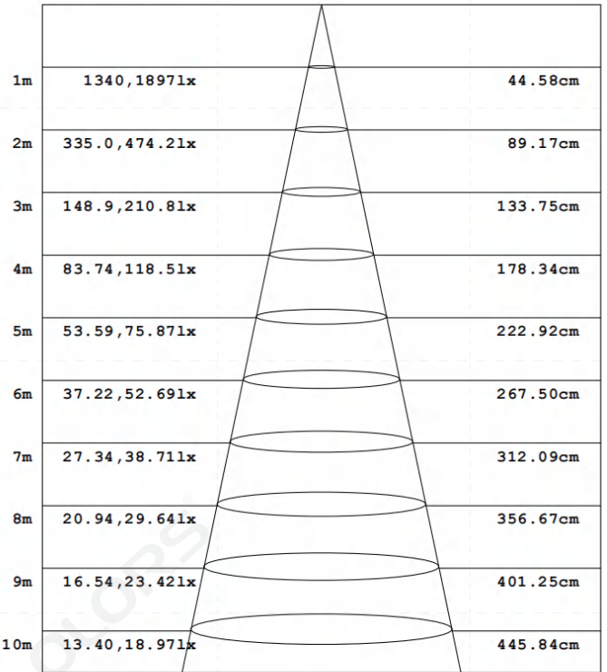
高度 Eavg, Emax 光束角: 25.13度 直径 注: 曲线为灯具在不同投射距离下的照射区域及区域内平均照度。 平均有效照度图
