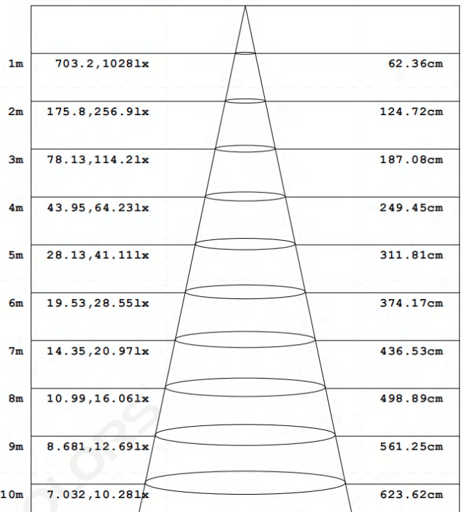
高度 Eavg, Emax 光束角: 34.64度 直径 注: 曲线为灯具在不同投射距离下的照射区域及区域内平均照度。 平均有效照度图
